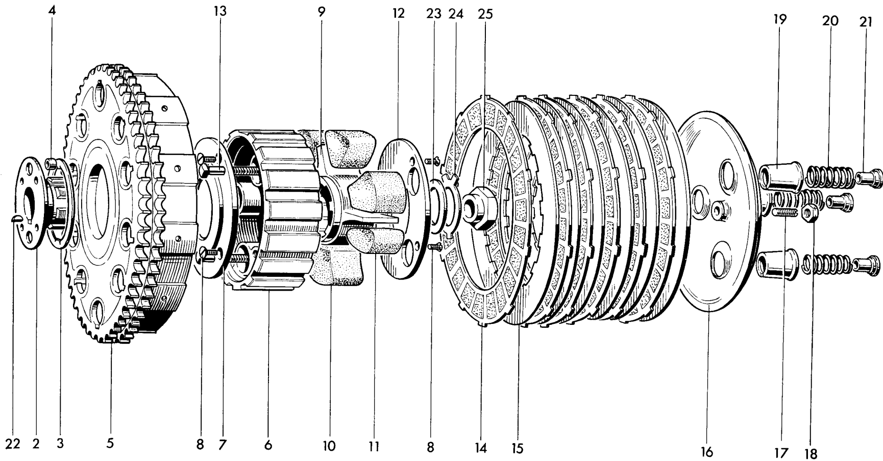
Fig. 10. CLUTCH
