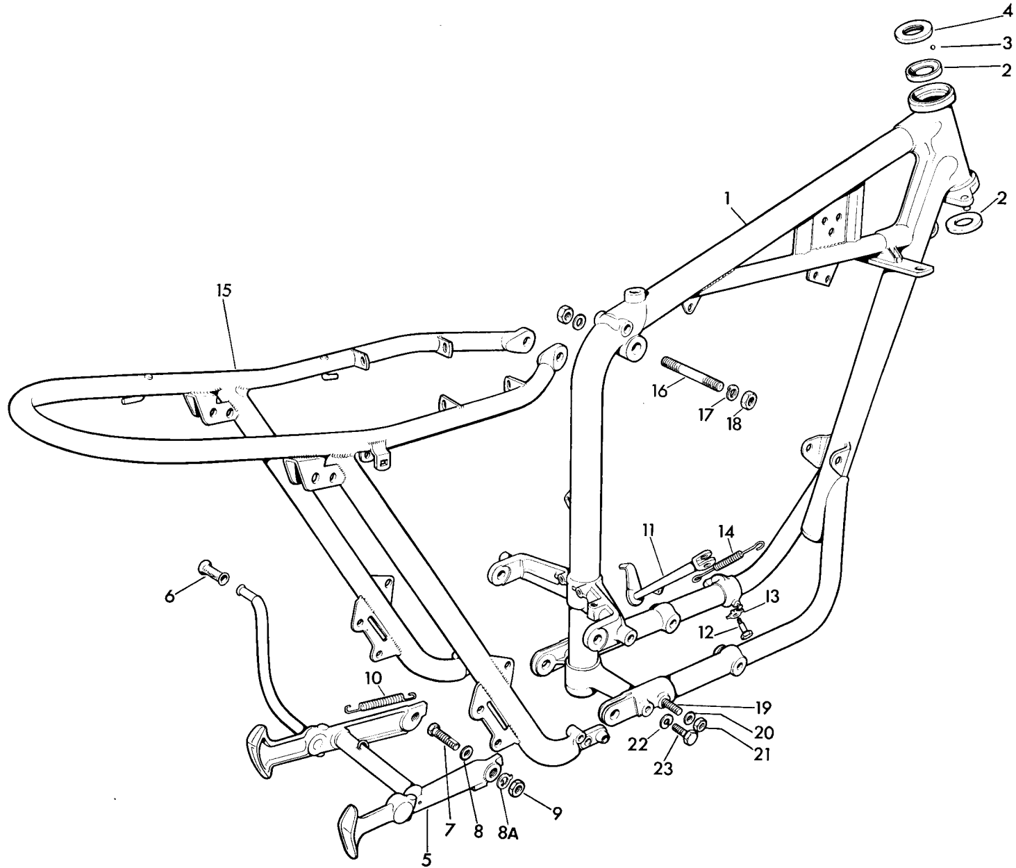
Fig. 12. FRAME
