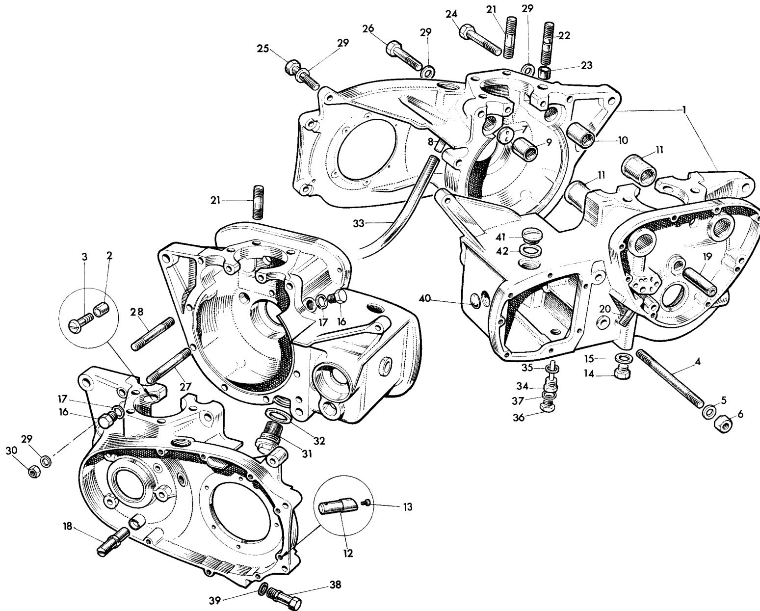
Fig. 2. CRANKCASE
