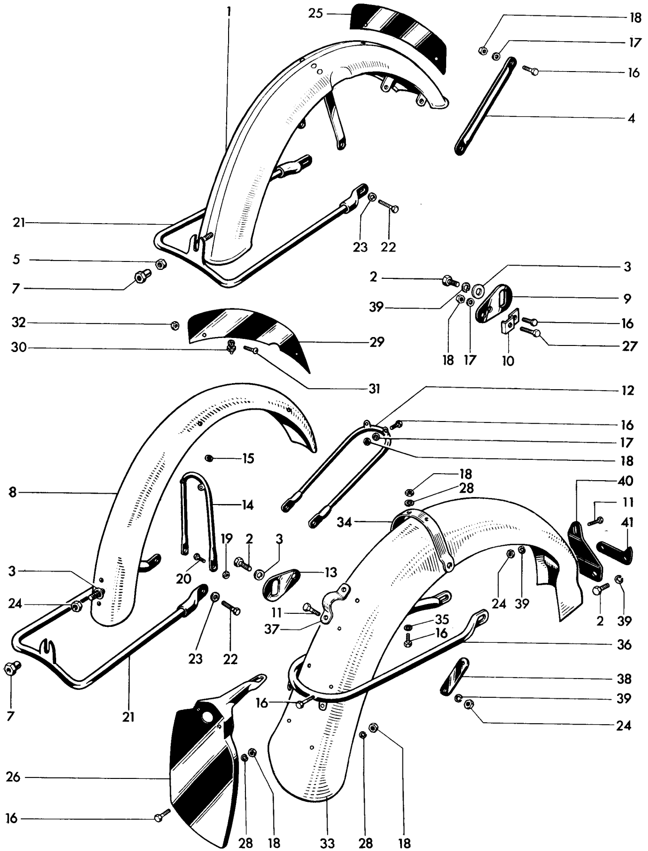
Fig. 26. MUDGUARDS
